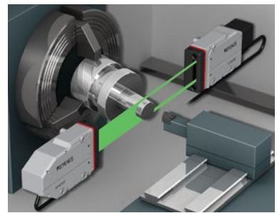
量測軸的外徑
